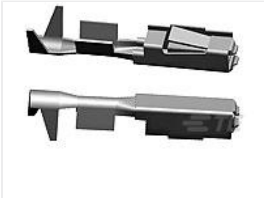
TE Part #144969-2 MOS0,63 Au rec LL unseal. 0,2-0,6
