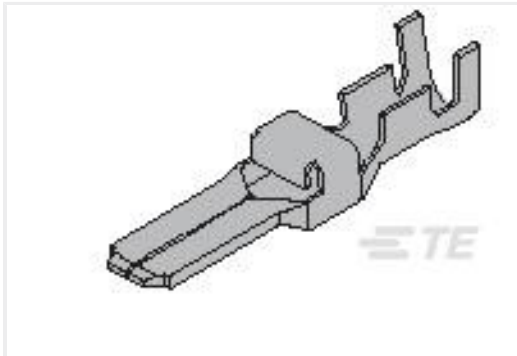
TE Part #84695-1 D5000 TAB CONT M LONG REEL AU PLATING
