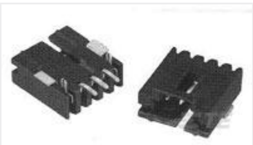
TE Part # 147278-3 04 MTE HDR SRRA SFMNT .100CL
