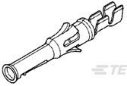
TE Part #66594-1 TYPE VI SKT CONT,MULTIMATE
