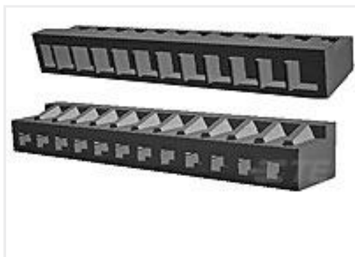
TE Part # 2-172520-3 LOW PRO MINI AMP IN 3P BLACK
