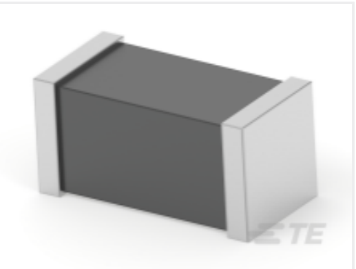
TE Part #2176496-1 BMC 0402 120R 25% A Med C
