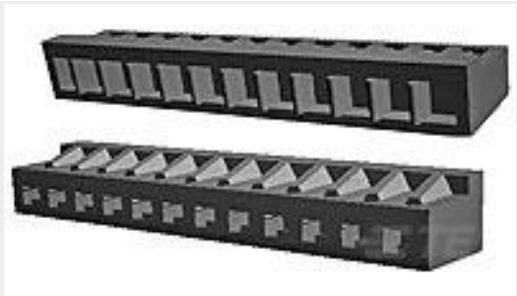
TE Part #172520-2 2P 2.5MM MINI AMP-IN HDR HSG
