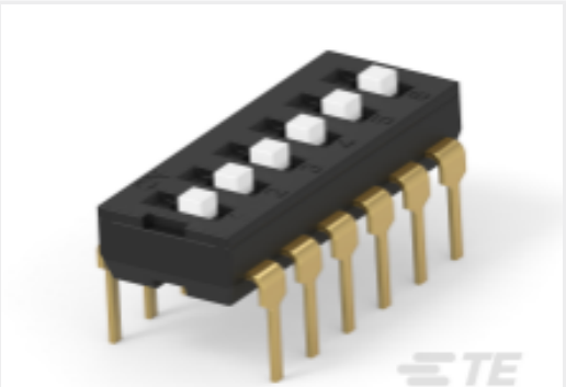
TE Part #2454982-4 ADE Next Gen. 06 Pos. THT TU
