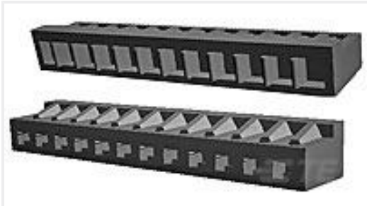
TE Part #172890-4 4P 2MM MINI AMP-IN HDR HSG
