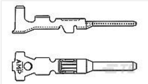
TE Part #282465-1 MINI MIC TAB CONTACT >1,5-
