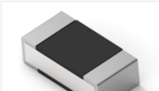
TE Part #1-2176313-5 RP 1E 0.1W 187K 0.1% 25PPM 1K RL
