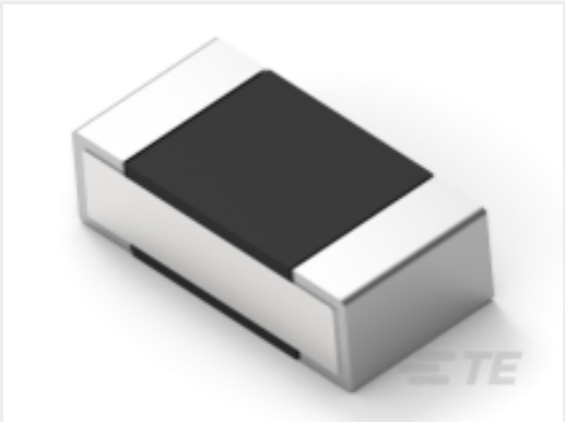
TE Part #2-2176308-5 RP 1E 0.1W 237K 0.1% 25PPM 5K RL
