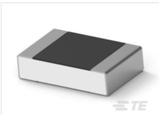
TE Part #6-2176373-8 RQ 0805 49R9 0.1% 10PPM 1K RL
