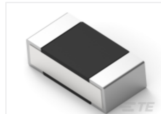
TE Part #9-2176305-8 RP 1E 0.1W 1K1 0.1% 25PPM 5K RL
