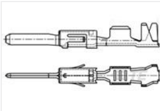
TE Part #963904-3 TAB A 1.6x0.6 CONTACT CS SWS Au
