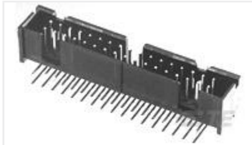
TE Part #103311-1 010 LOPRO HDR RA 30DP
