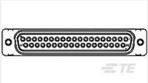
TE Part #1484948-1 AMPLIMITE,PLG ASY,37P,SZ4,SER109
