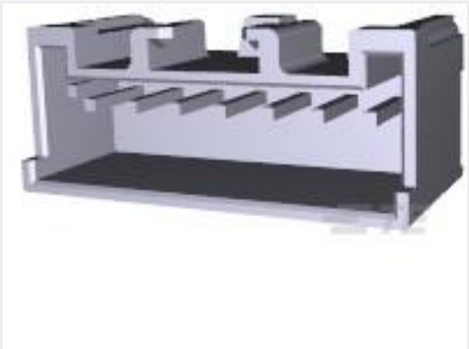
TE Part #917785-1 2.5 S.D.L POST HDR ASY 7P STD
