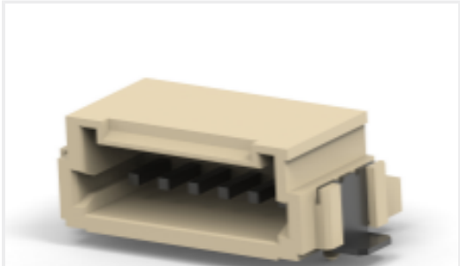
TE Part # 292227-6 1.5 MINI CT SGL H SMT W BOSS 6
