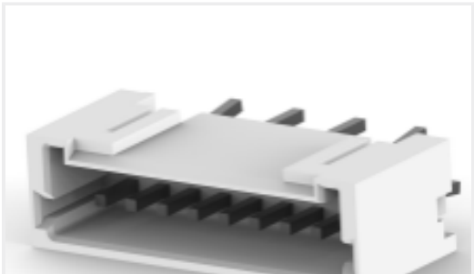
TE Part # 2-292207-9 MINI CT SGL DIP V 9P BLACK
