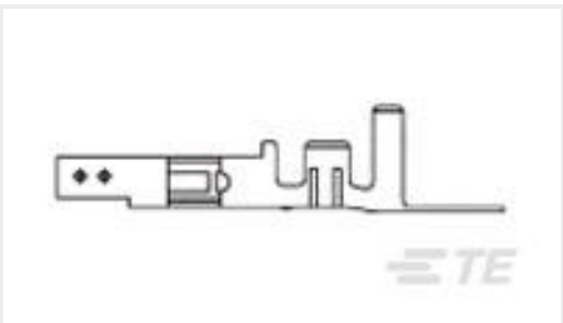
TE Part #794958-3 VAL-U-LOK SKT PHBZ SN 22-26AWG
