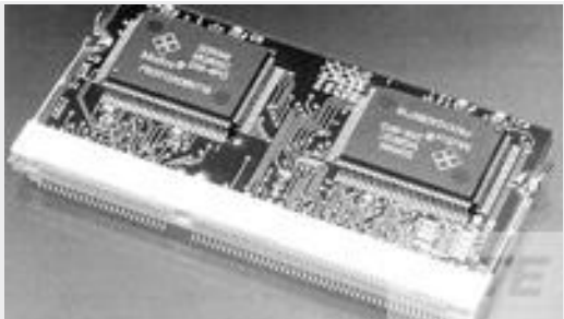
TE Part #6-390112-1 SKT,SODIMM,144P,SDRAM3.3V,HIGH, T&R
