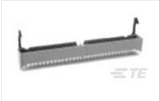
TE Part #3-1761713-3 IDC LOW PRO HDR 40P VERT SHT L
