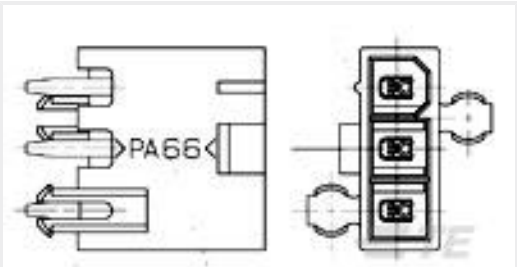
TE Part #2029058-3 3P VAL-U-LOK SR HDR SN V2 WODH
