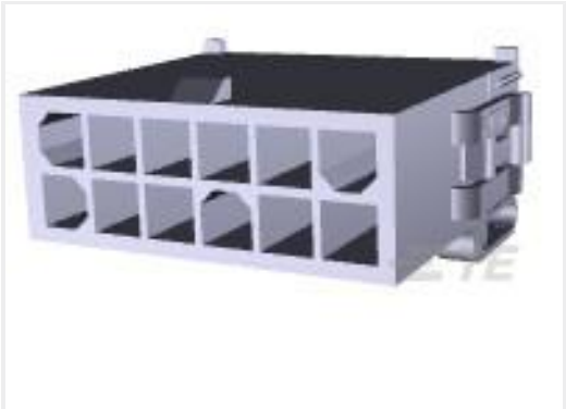
TE Part #794199-1 12P MINI UMNL2 CAP HSG DBLROW
