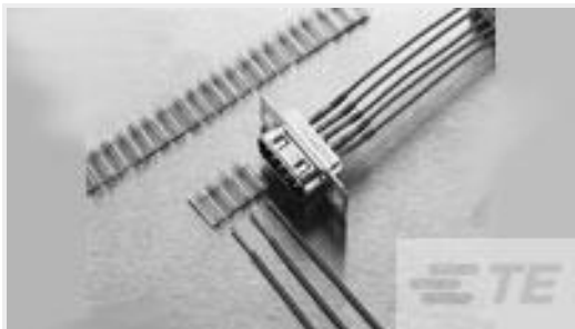
TE Part #626152-000 D-704-0043
