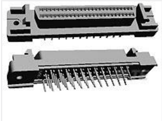
TE Part #5749069-9 100 50SR VERT RCPT ASSYY
