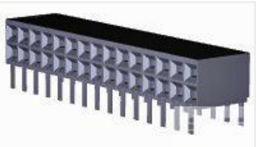
TE Part #2-5535512-2 30 MODII HORZ DR CE EESS .100
