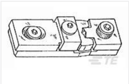
TE Part #59828-1 TETRA-CRIMP DIE 12-10
