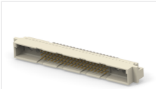
TE Part #374169-E STVM 60-4 M ABC VVV 4-00 0606 ** 137 E0
