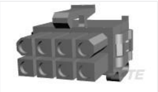
TE Part #794245-1 08P MINI UMN L2 PLUG HSG UL94V2
