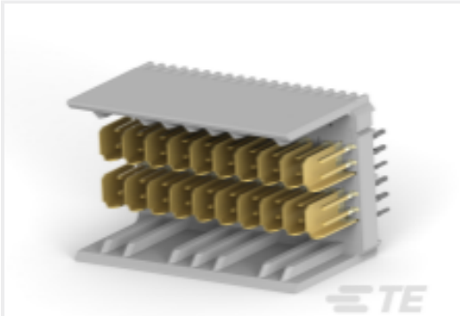
TE Part # 1469025-1 HM-ZD 2PR HDR 40P 2.5MM
