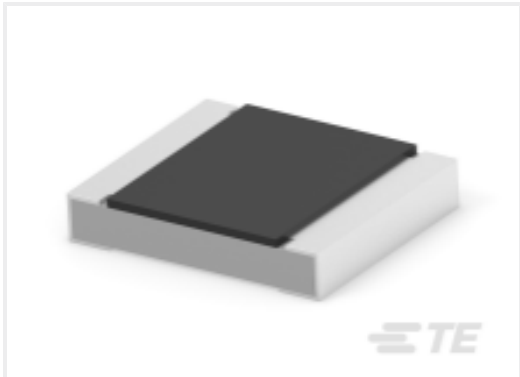
TE Part #5-2176587-4 RLC73K 2E R20 1% 1K RL
