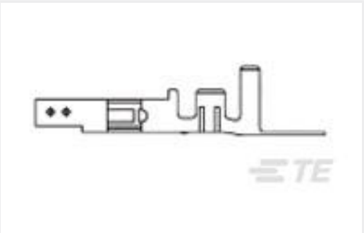
TE Part #794956-4 VAL-U-LOK SKT PHBZ AU 22-18AWG
