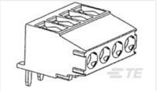
TE Part #284415-2 TERMI-BLOK 900 PCB 2 POS. 3,81
