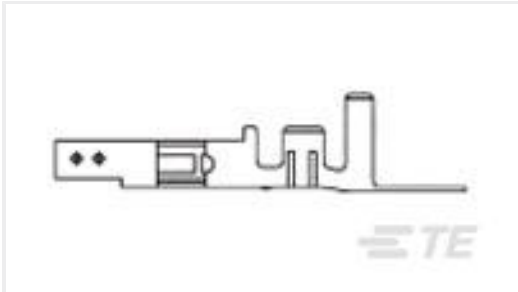
TE Part #1586315-3 VAL-U-LOK SKT PHBZ SN 24-18 LP
