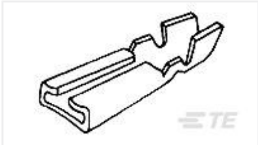
TE Part #42765-1 TAPER TAB 078 REVERSE REEL REC 24-22TPBR
