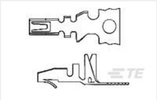
TE Part #3-794121-1 TERMINAL, MINI AMP-IN 2000 22-18 AWG
