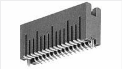
TE Part #5-292227-3 1.5 MINI CT SGL H SMT W BOSS 3
