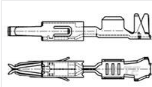
TE Part #4-1241732-1 MT3 REC 1.6 Contact SRC Au
