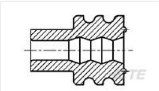
TE Part #963292-1 WIRE SEALING 2,2
