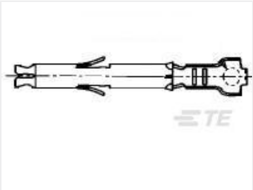
TE Part #170366-3 MINI UNIVERSAL M-N-L SOCKET LP
