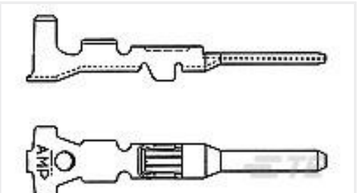
TE Part #282109-3 MINI MIC TAB CONTACT
