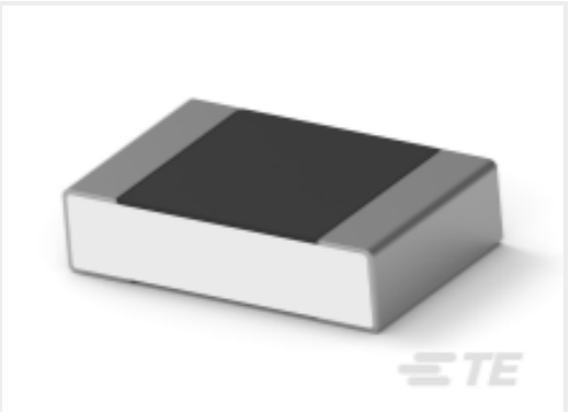
TE Part #4-2176381-3 RQ 0805 34K 0.1% 10PPM 5K RL
