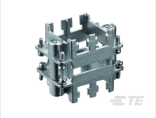
TE Part #T2070164201-000 H16BN-T4-F
