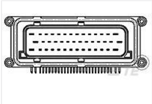
TE Part #1-963484-1 MESSERLEISTE MIX70P
